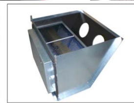
空調ダクト内バス用光線ストリーマ除菌ユニット
